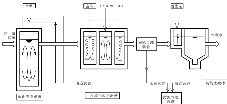
図4.5.4(3) 基本フローシート（高負荷脱窒素処理方式）
