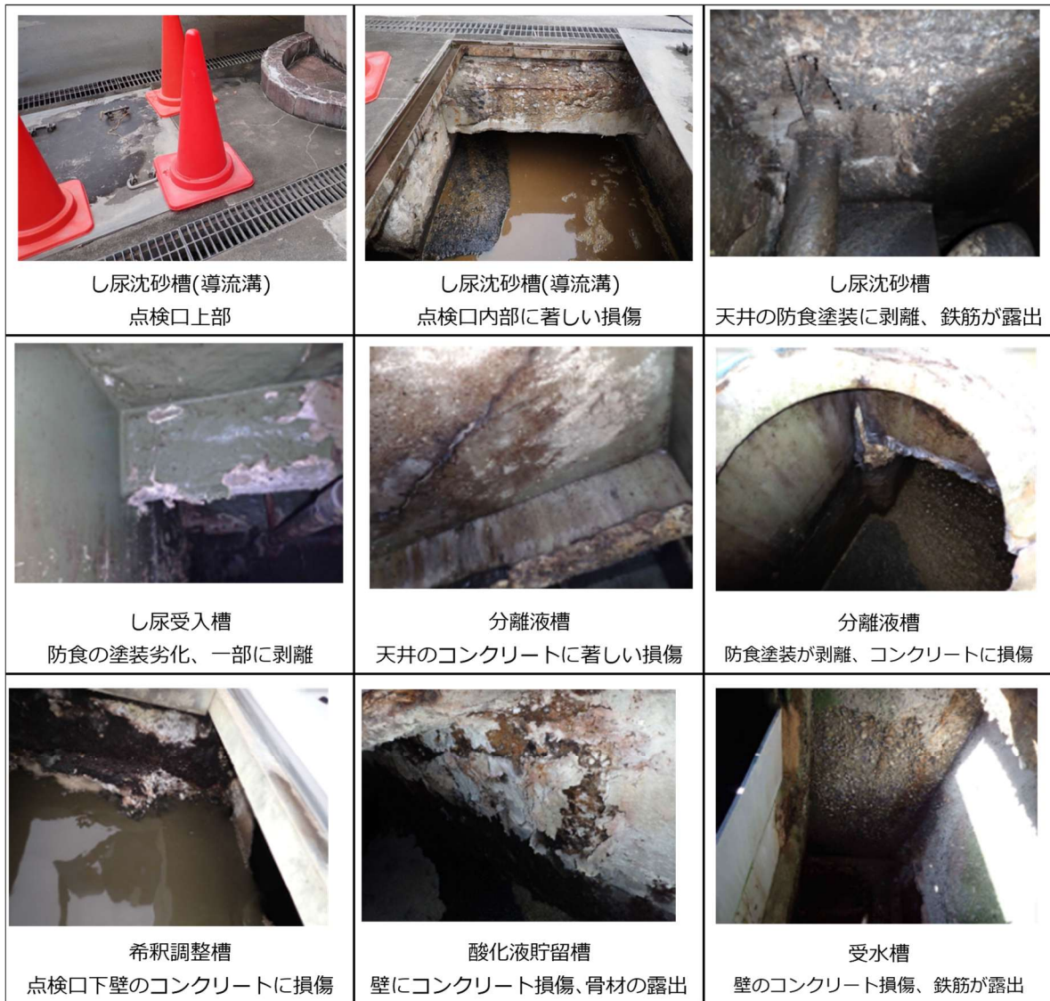
図1.3.1 早期に対応が必要なRC水槽
