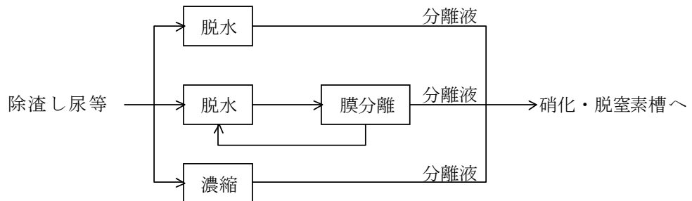
図4.5.11 前凝集分離設備の分類
