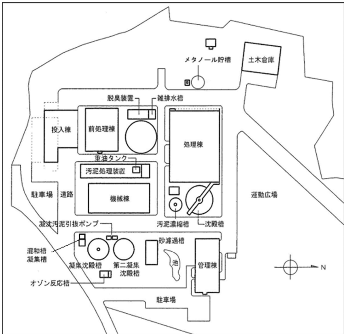
図1.1.4 全体配置図
