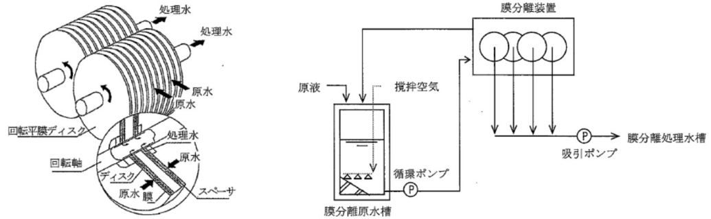
図4.5.8 回転平膜
