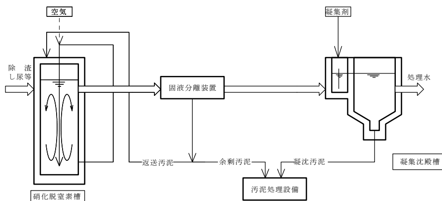
図4.5.4(2) 基本フローシート（高負荷脱窒素処理方式）
