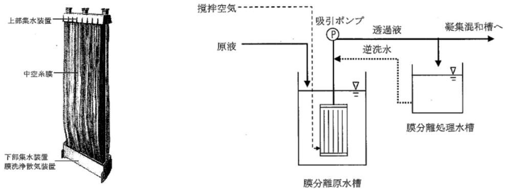
図4.5.9 中空糸膜
