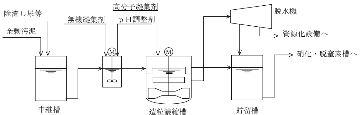
図4.5.12(2) 前脱水分離方式のフロー例
