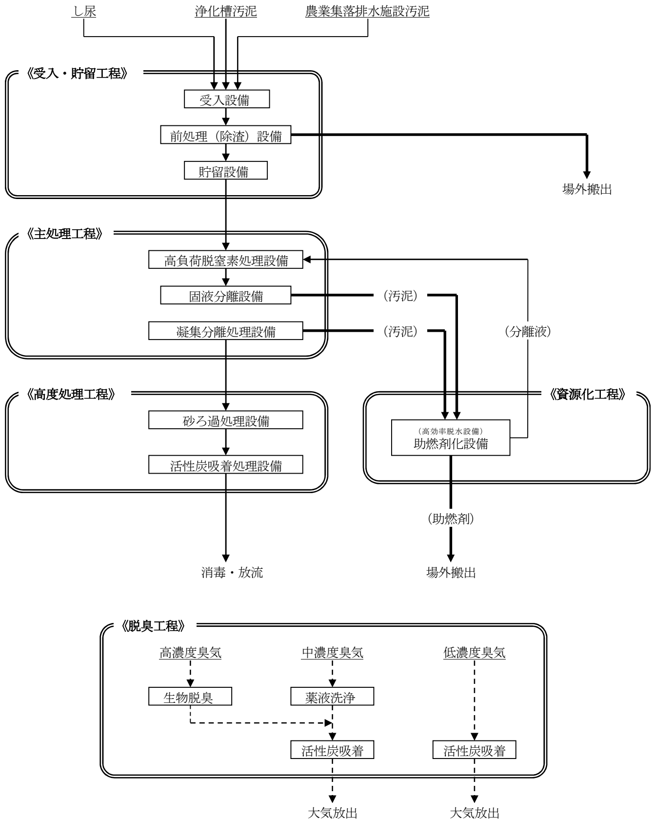
図6.1.1(1) 計画施設の基本フローシート(高負荷脱窒素処理方式)
