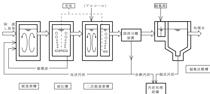
図4.5.4(1) 基本フローシート（高負荷脱窒素処理方式）
